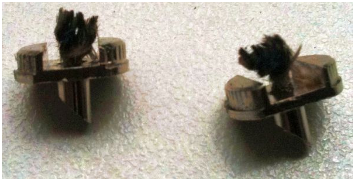
Verkohlte Faser verursacht durch Liquidmangel.
